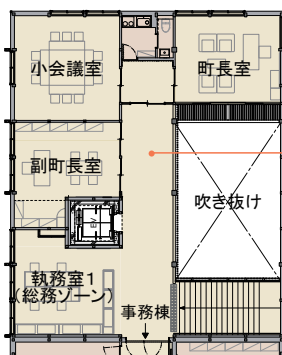
● 2階平面図
