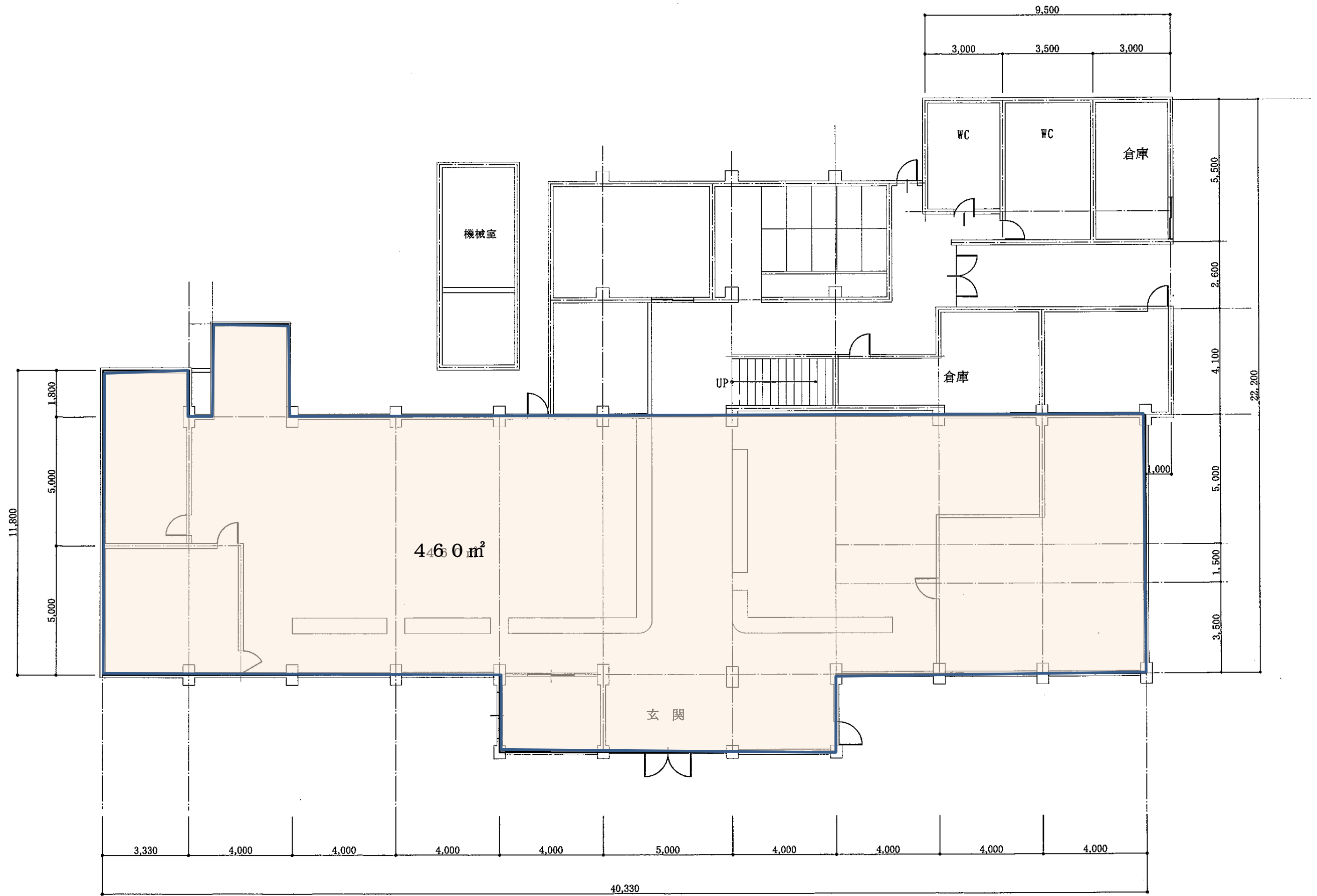
宮之浦支所庁舎1階平面図
