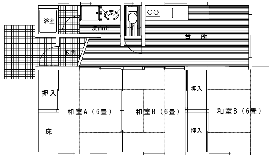
本図面は12号の平面図 14号は反転配置。
