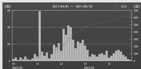
火山性地震の daily 地震回数と積算回数 (令和3年4月1日~5月20日)
