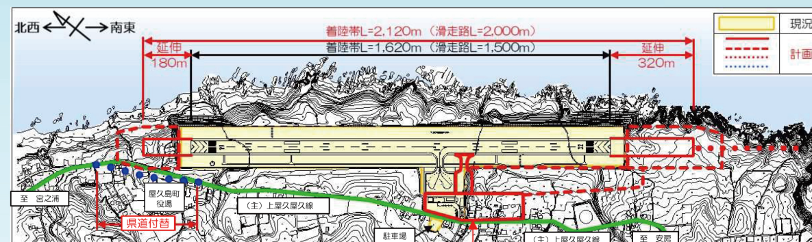
基本計画図
