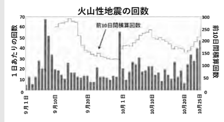
▲火山性地震の日別回数と前10日間積算回数(2023年9月1日～10月25日)
