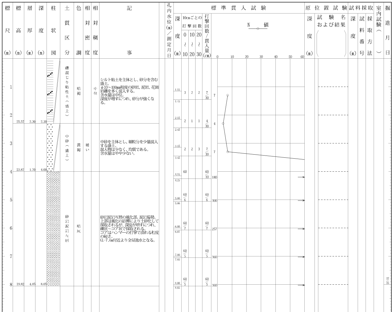
図 3-2-3 ボーリング柱状図 (調査 No.1)
