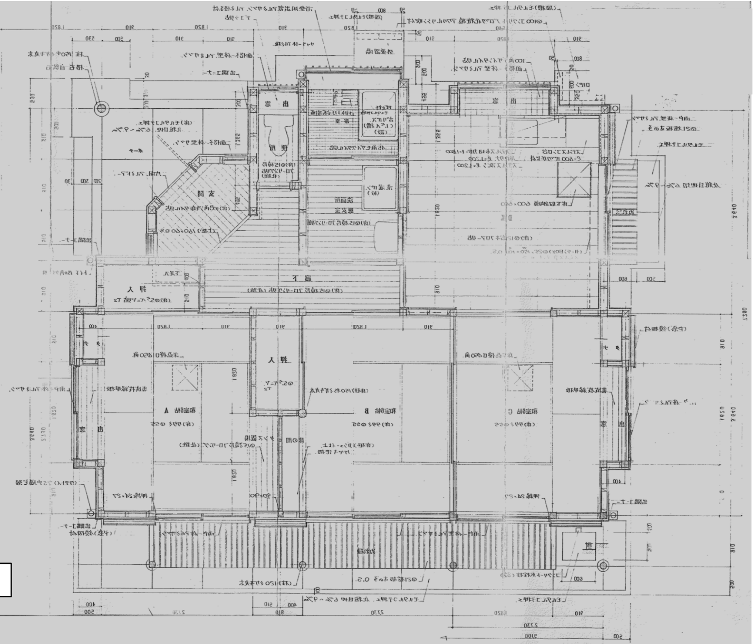
6号棟 平面図
